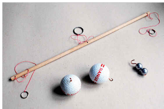
Obr. 1 – rovnoramenné váhy s příslušenstvím
