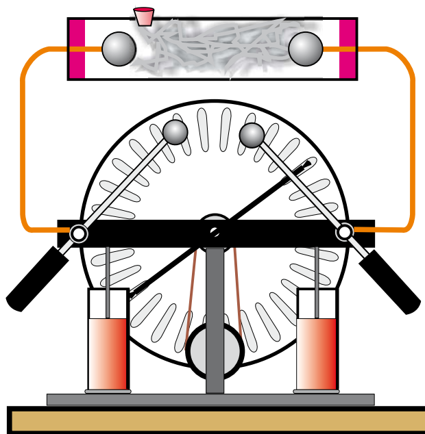
Obr. 34 – princip elektrostatičkého odlučovače popílku
