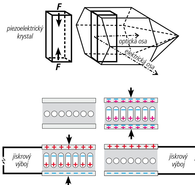
Obr. 30 – princip činnosti piezoelektrického zapalovače
