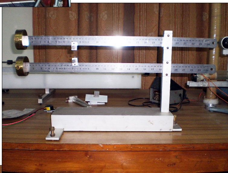
Obr. 14 – magneticky sprzęžené oscilátory
